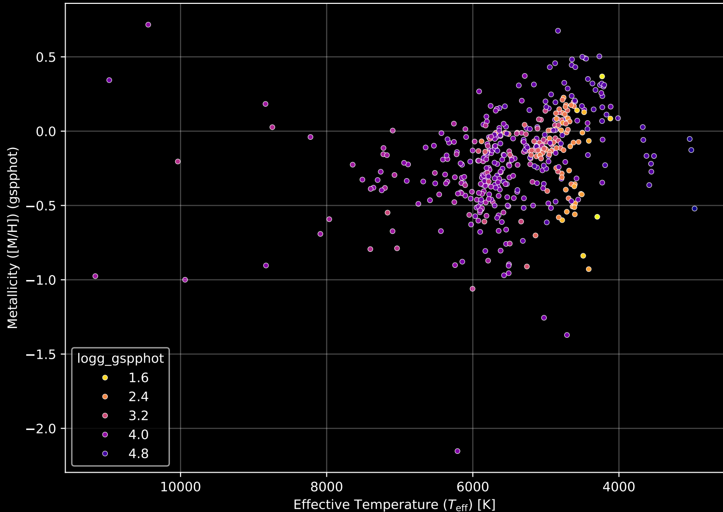
APOGEE DR17 Field: [N188] Stellar Population Parameters (n= 455)
